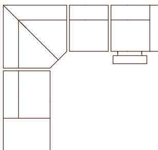
1.5EHR (1ARM&RHF) - 1.5S NO ARM - CORNER - ONE END CHAISE (LHF) 236cm (W) 292cm (D)
